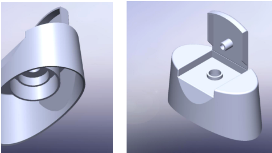
VISTA ISOMETRICA
